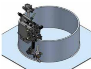
Corte/Soldadura circular
