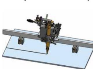
Corte recto
